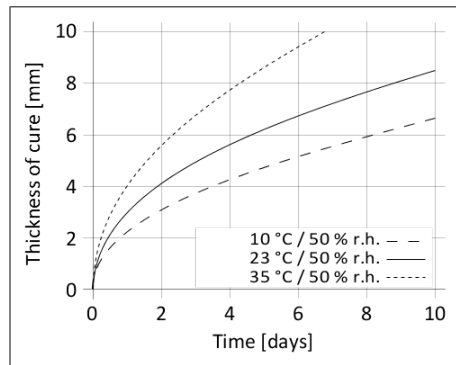
Schema 1: Uithardingssnelheid Sikaflex®-554
